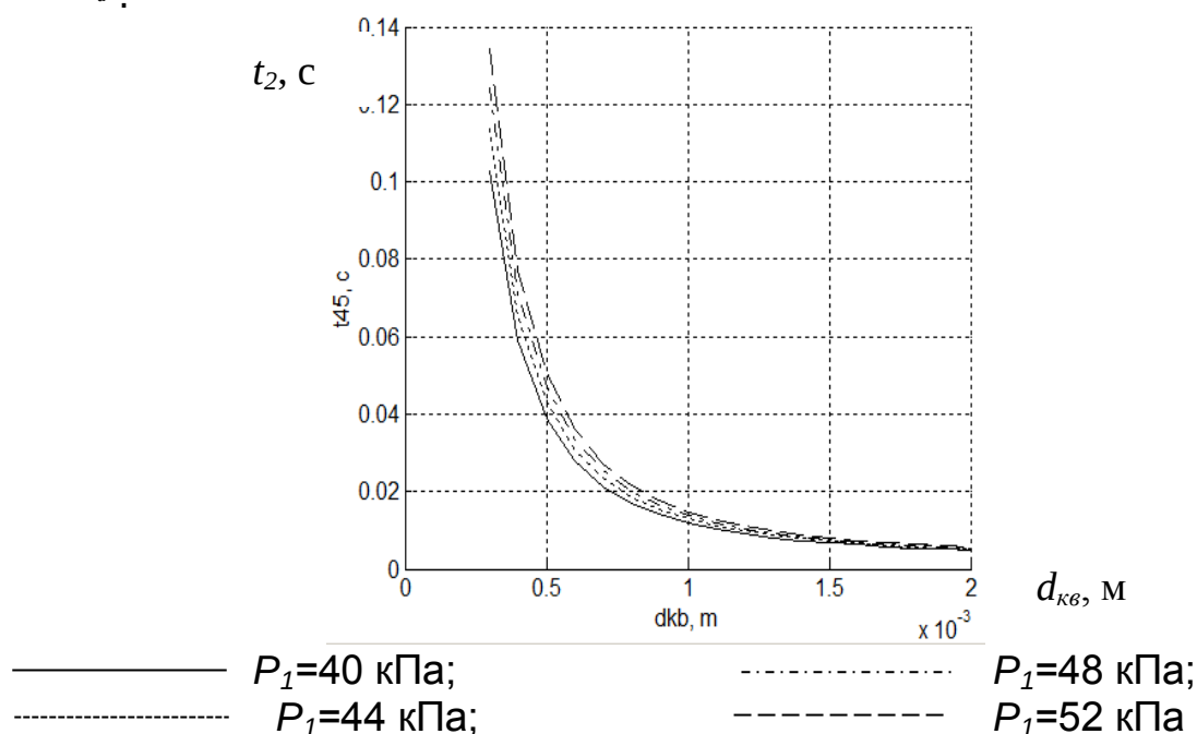
Рис. 2. Залежність тривалості часової затримки завершення руху клапанів від діаметра каліброваного отвору при переході пульсатора від такту ссання до стиску.
