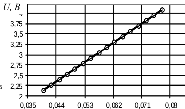
Рис. 3. Калібрувальні графіки зміни вихідної напруги U тензодавачів вимірювачів потоку сипучих матеріалів від маси m_K кожного потоку по тензовимірювальній площині (а) від 2,0 до 75,5 г/с і (б) від 75,0 до 545,5 г/с.
