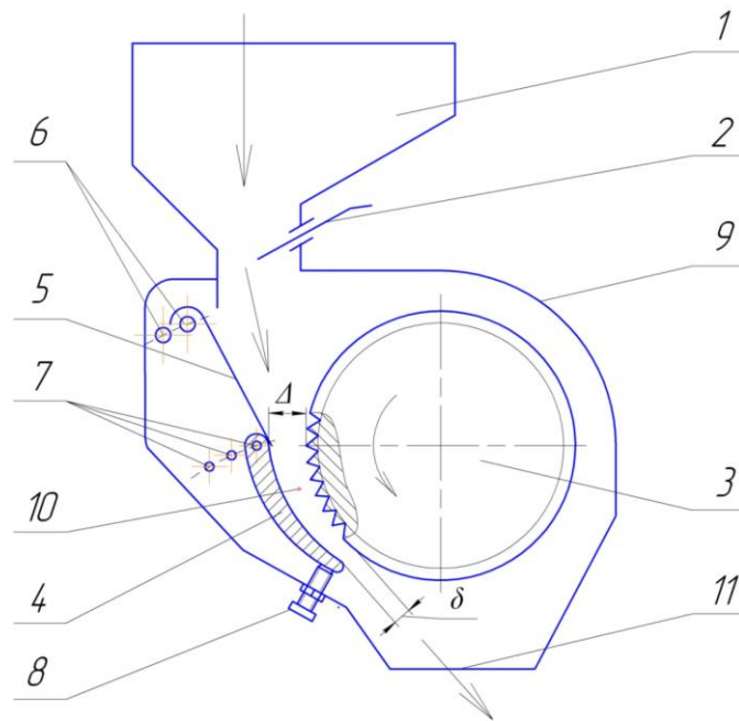
Рис. 1. Конструктивно-функціональна схема дробарки: 1 – зерновий бункер; 2 – регулювальна заслінка; 3 – валець; 4 – дека; 5 – напрямна; 6, 7 – кріплення відповідно напрямної та деки; 8 – регулювальний гвинт; 9 – корпус; 10 – робоча зона; 11 – вивантажувальне вікно.
