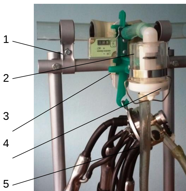
Рис. 6. Загальний вигляд автономного модуля у складі доїльного апарату: 1 – фрагмент молоко провідної лінії з краном; 2 – протоchnий датчик ємнісного типу; 3 – автономний модуль з цифровим індикатором; 4 – дозуючий пристрій; 5 – підвісна частина доїльного апарату.
