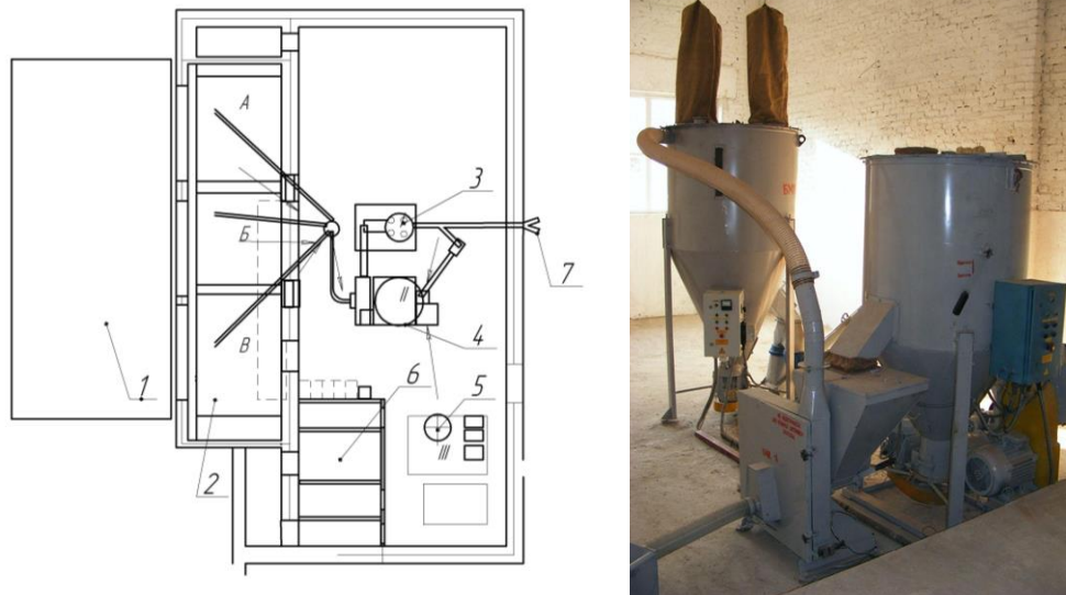
Рис. 3. Ситуаційний проект розміщення обладнання комбікормового агрегату та загальний його вид: 1 – під'їзний майданчик; 2 – накопичувачі зернових компонентів ( 3\text{--}5\text{ м}^3 ); 3 – основний змішувач ( 1,2\text{ м}^3 ); 4 – змішувач добавок ( 0,2\text{ м}^3 ); 5 – змішувач блендів ( 0,01\text{ м}^3 ); накопичувачі добавок; 7 – готовий комбікорм.
