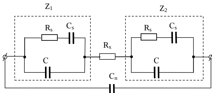
Рис. 1. Еквівалентна схема двоелектродної кондуктометричної комірки.
