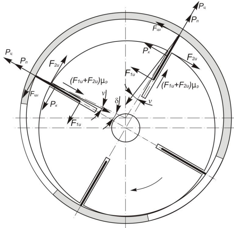
Рис. 1. Схема розподілу навантажень від сили інерції, що діє на радіальну пластину.
