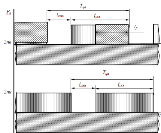
Рис. 4. Індикаторна діаграма роботи пульсатора: - в міжстіно- нкій камері доїльного стакана; - в піддійковій камері доїльного стакана; - ділянка діаграми де можливе регулювання співвідно- шення тактів у веденій секції пульсатора.
