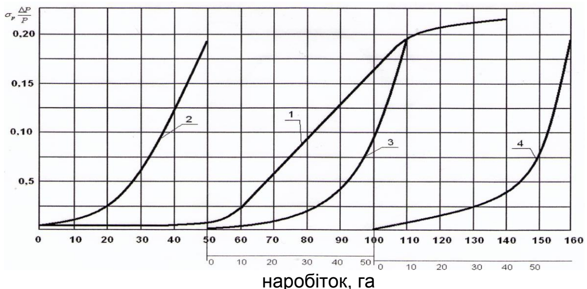
Рис. 4. Відносний знос за масою серійного та зміцненого лемішів: 1 – леміш з точковим зміцненням; 2 – серійний леміш (перша установка); 3 – серійний леміш (друга установка); 4 – серійний леміш (третя установка).
