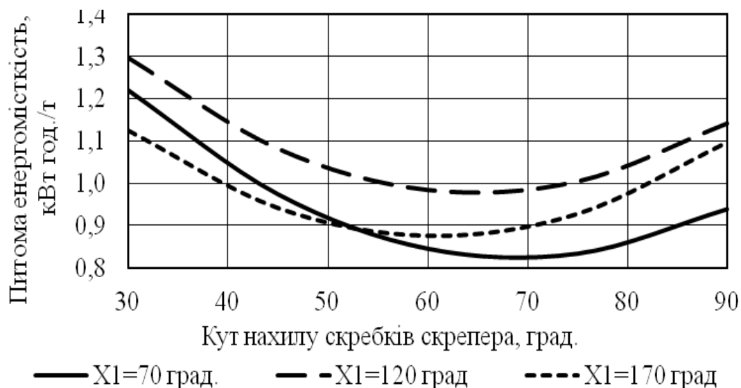
Рис. 6. Залежність питомої енергомiсткостi удосконаленої скреперної установки вiд кута нахилу скребкiв скрепера.
