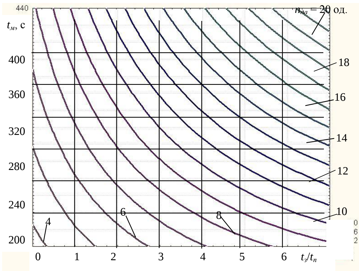
Рис. 3. Графік проєкції поверхні відгуку залежності кількості доїльних апаратів n_{da} , що обслужить ОМД від тривалості машинного доїння t_M корови і співвідношення завершальних і підготовчих операції t_3/t_n .
