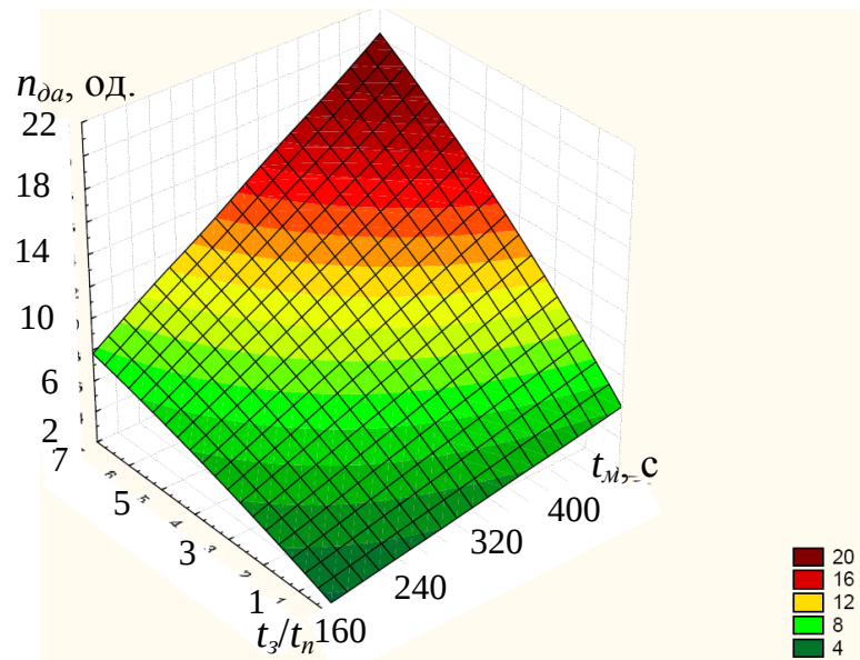
Рис. 2. Залежність кількості доїльних апаратів n_{da} , що обслужить ОМД від тривалості машинного доїння t_M корови і співвідношення завершальних і підготовчих операції t_3/t_n .
