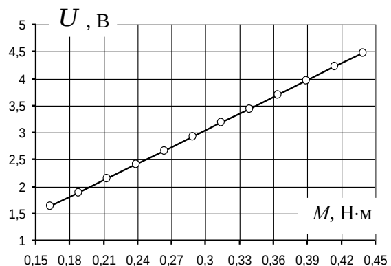
Рис. 4. Калібрувальні графіки зміни вихідної напруги U тензодавачів вимірювача крутного моменту від зміни зусилля крутного моменту M для витрат потужності (а) від 10 \cdot 10^{-3} до 1,0 Вт і (б) від 1,0 до 7,0 Вт.
