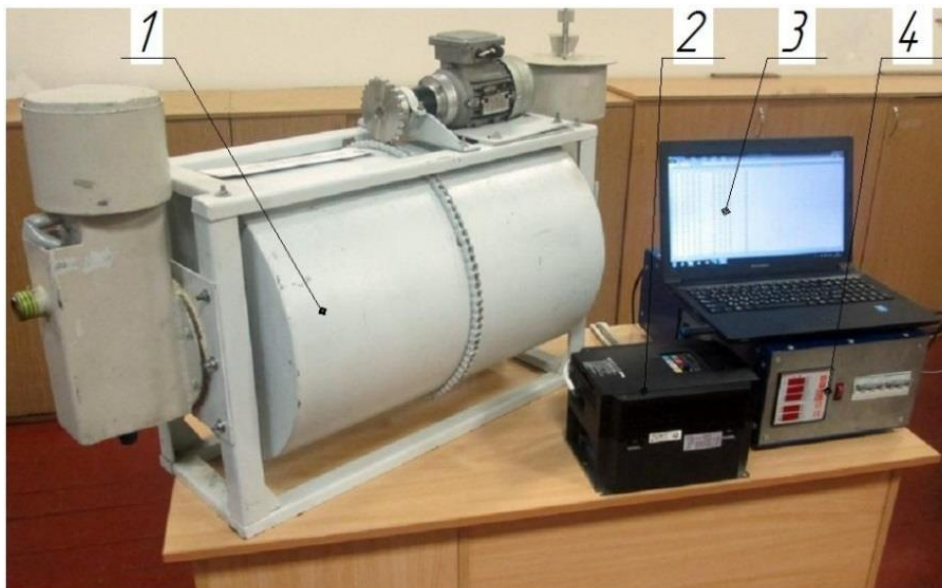
Рис. 1. Комплект обладнання для проведення для дослідження енергетичної ефективності перемішування субстрату (зовнішній корпус не показано): 1 – обертний метантенк, 2 – частотний перетворювач, 3 – реєстратор, 4 – цифровий вимірювальний пристрій.
