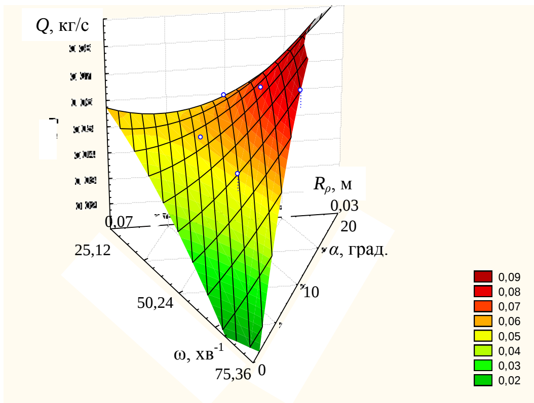
Рис. 3. Залежність продуктивності Q дозатора-змішувача компонента, що вводиться від кутової частоти \omega обертання диска, кута твірної \alpha дозуючого диска і радіуса кривизни R_\rho лопаток диска при вакуумметричному тиску P_e=3 кПа.
