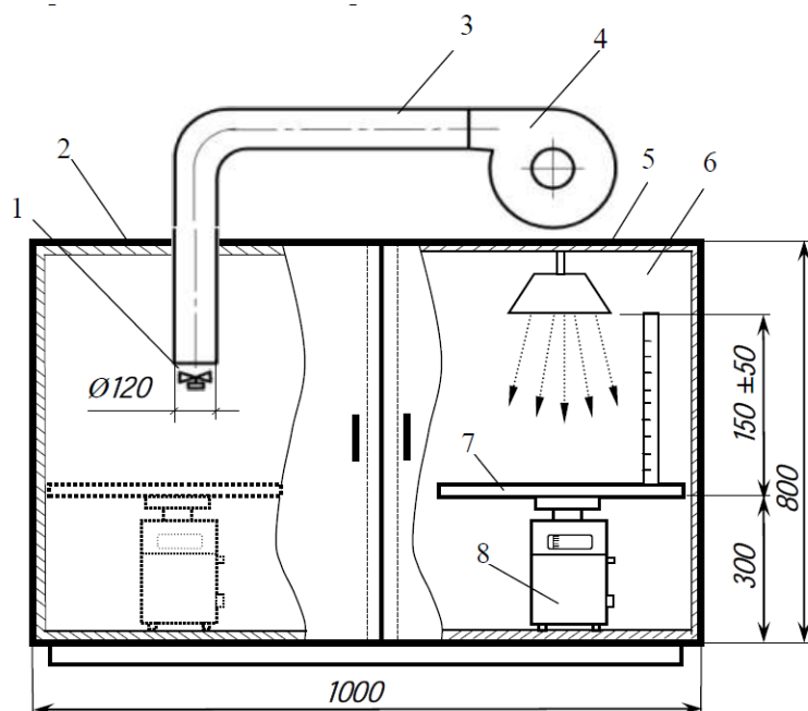
Рис. 1. Схема лабораторної установки для визначення раціональних параметрів перервного ІЧ-сушіння: 1 – анемометр АПР2; 2 – камера відлежування; 3 – повітропровід; 4 – тепловентилятор; 5 – ІЧ-випромінювач; 6 – камера опромінювання; 7 – підставка з об'єктом сушіння; 8 – терези.
