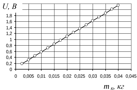
Рис. 3. Калібрувальні графіки зміни вихідної напруги U тензодавачів вимірювачів потоку сипучих матеріалів від маси m_K кожного потоку по тензовимірювальній площині (а) від 2,0 до 75,5 г/с і (б) від 75,0 до 545,5 г/с.
