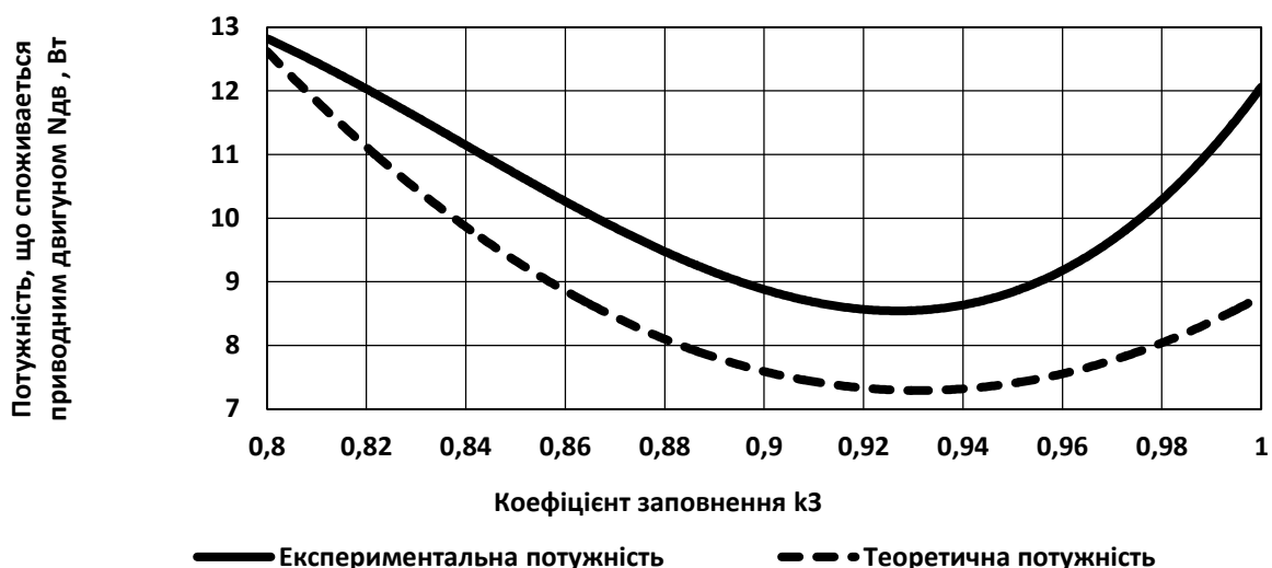
Рис. 3. Дослідна та теоретична залежності потужності електро-двигуна N_{\partial\partial} , для забезпечення обертання біореактора від коефіцієнту заповнення k_3 (внутрішній радіус R=0,2 м, робоча довжина L=0,6 м, кутова швидкість \omega=0,11 рад/с) при коефіцієнті занурення k_{3H}=1 .
