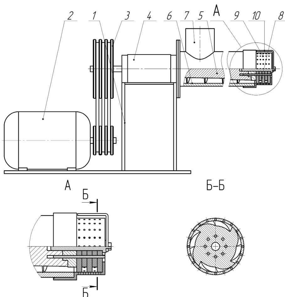
Рис. 1. Конструктивно-технологічна схема установки для виготовлення пелет (пелетератора).
