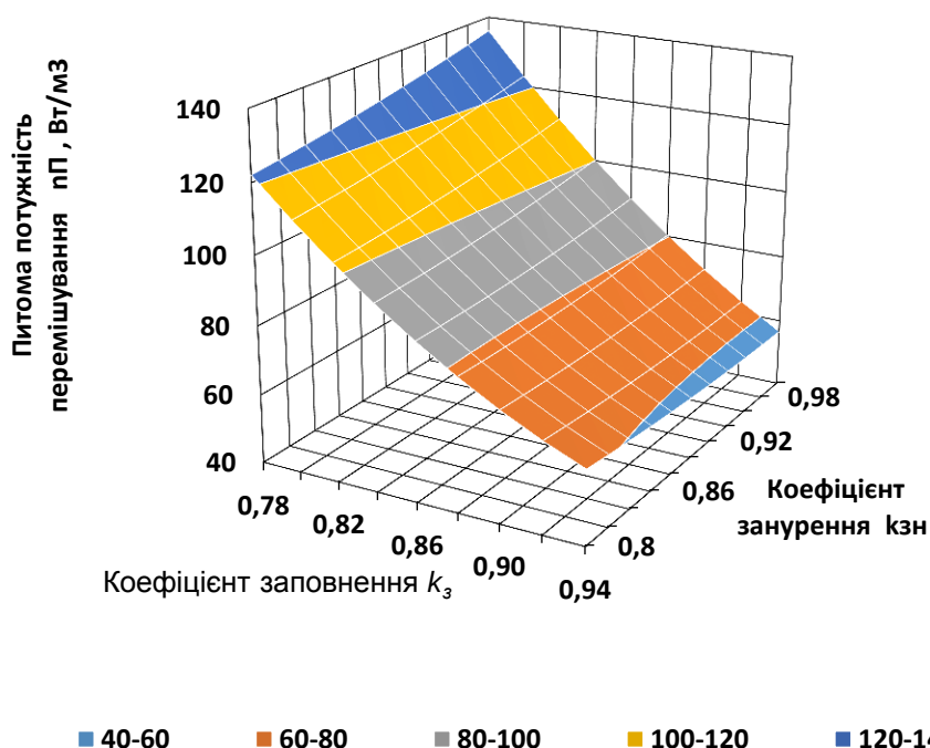
Рис. 4. Залежність питомої потужності n_{\Pi} перемішування біомаси в реакторі від коефіцієнтів заповнення k_z та занурення k_{zn} (внутрішній радіус R=0,2 м, робоча довжина L=0,6 м, кутова швидкість \omega=0,11 рад/с).
