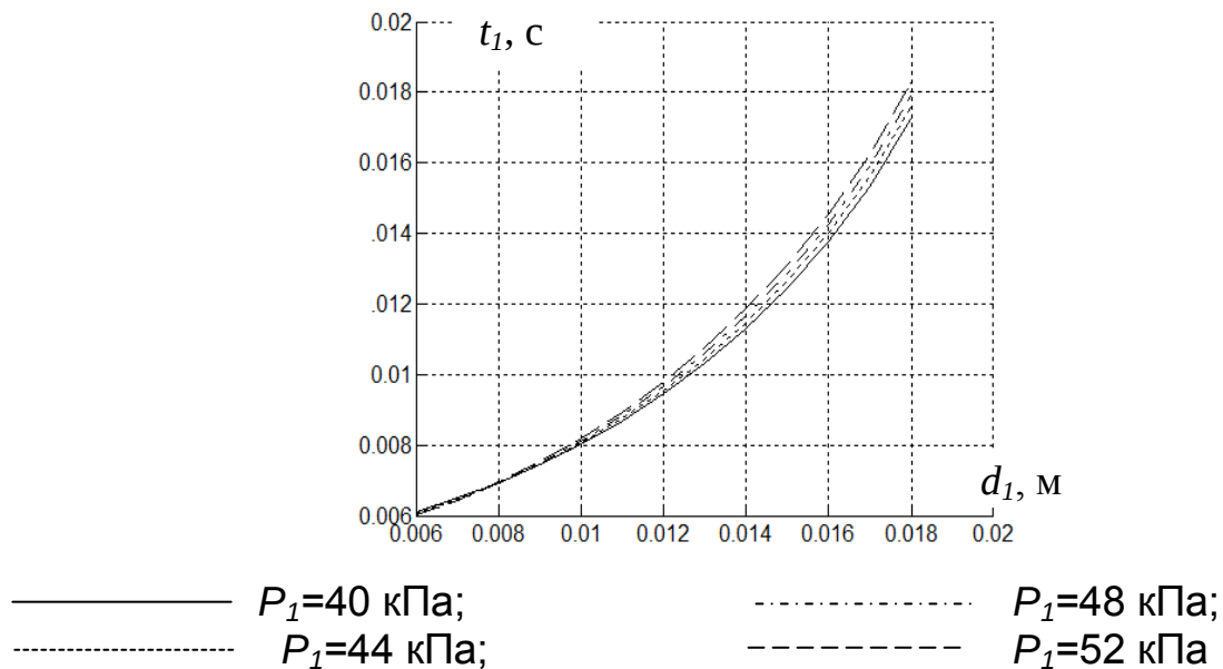
Рис. 1. Залежність тривалості часової затримки завершення руху клапанів від діаметра верхнього перепускного отвору при переході пульсатора від такту стиску до ссання.
