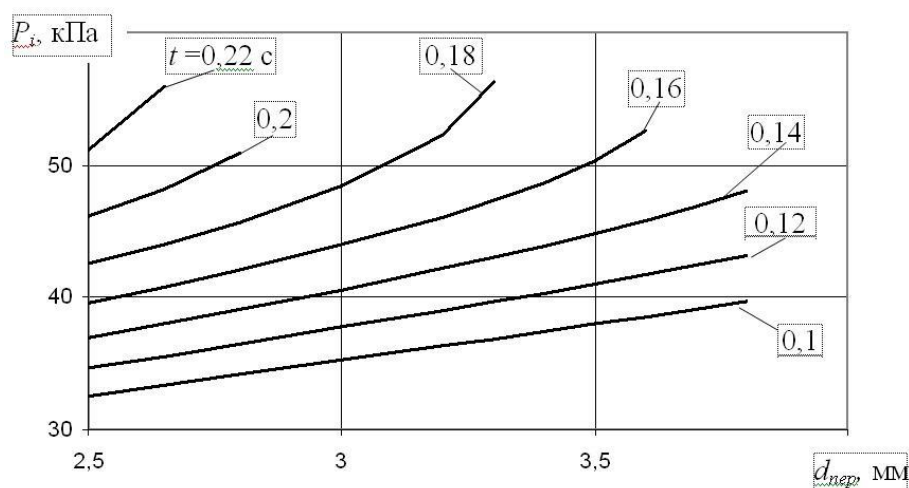
Рис. 2. Вплив вакуумметричного тиску P_i від діаметра d_{пер} перепускного отвору на тривалість t наповнення повітрям камер змінного вакуумметричного тиску системи “доїльний стакан – пульсатор”.
